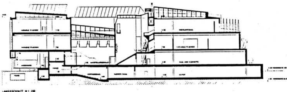
Längsschnitt
